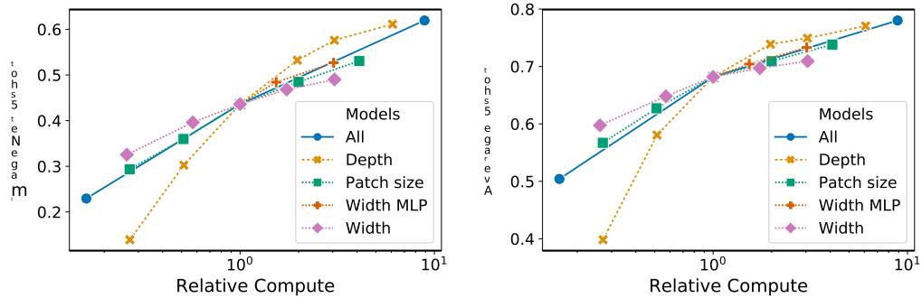
图8: 缩放视觉Transformer的不同模型维度。
